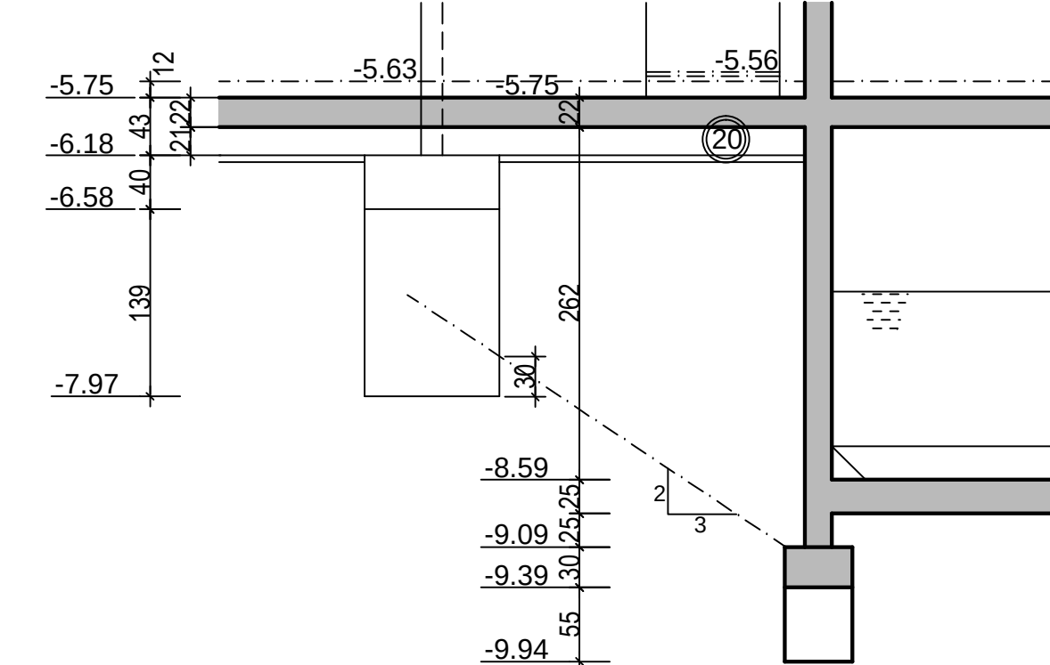
COUPE 2 Ech: 1/50
