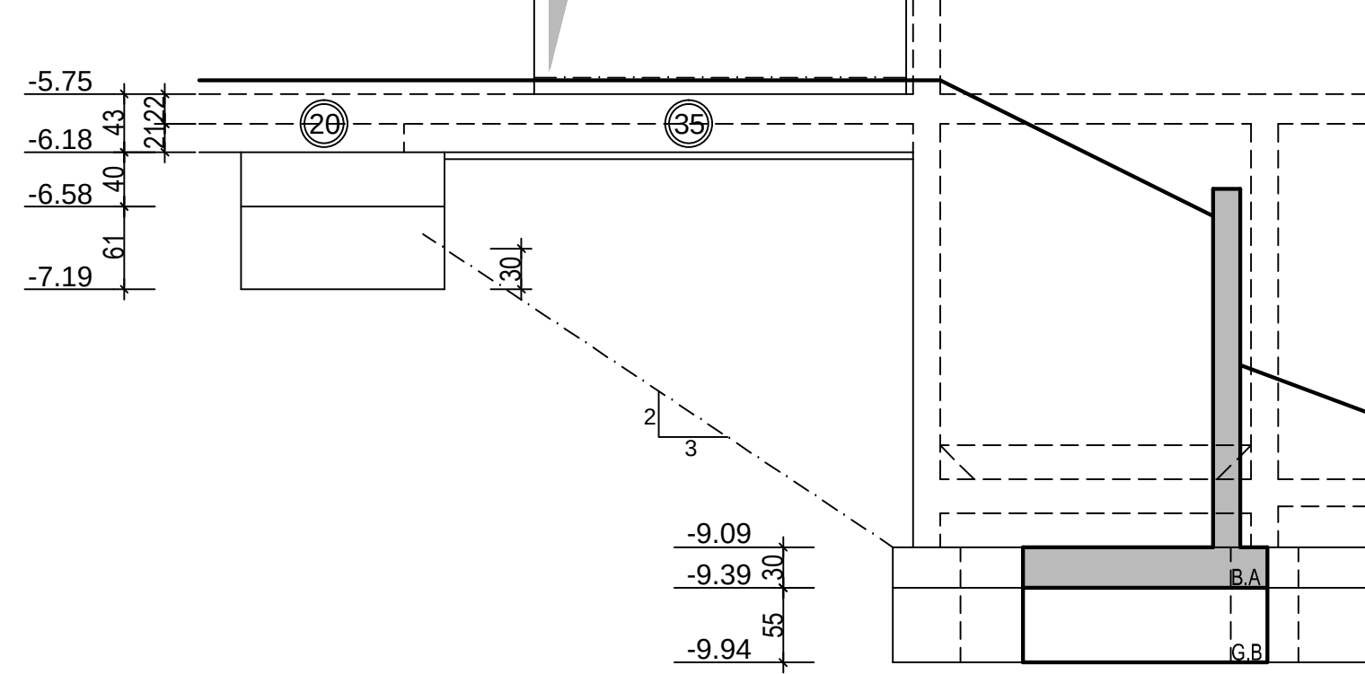
COUPE 1 Ech: 1/50
