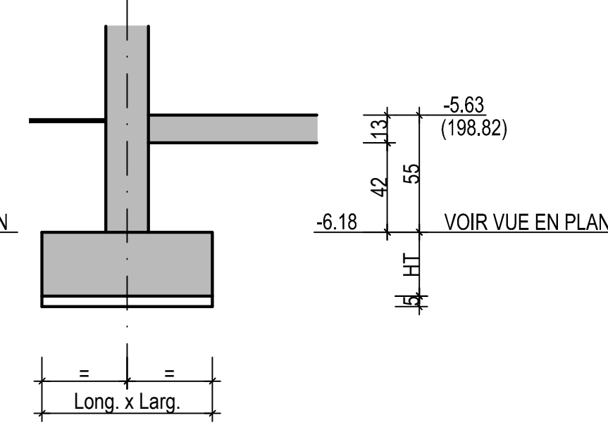
COUPE SUR DALLAGE
