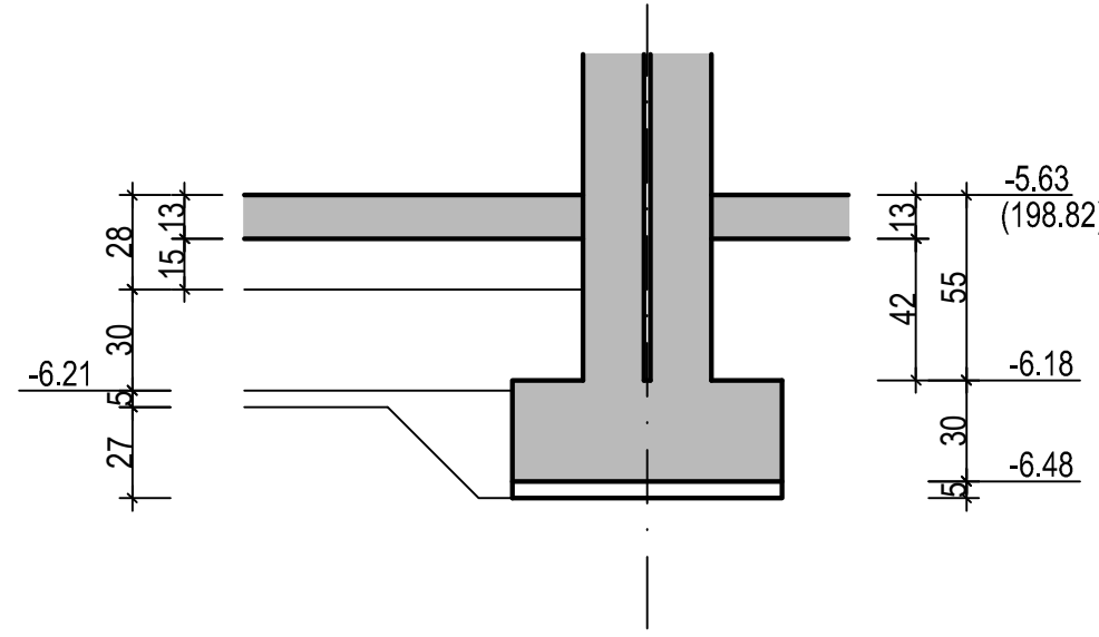
COUPE A Ech: 1/25
