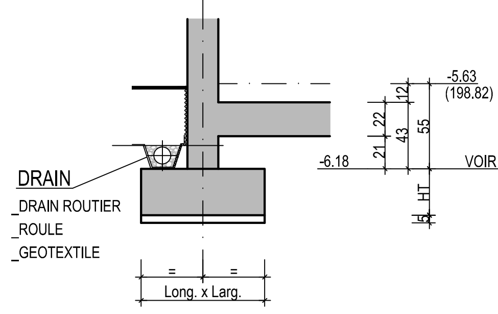
COUPE SUR DALLE
