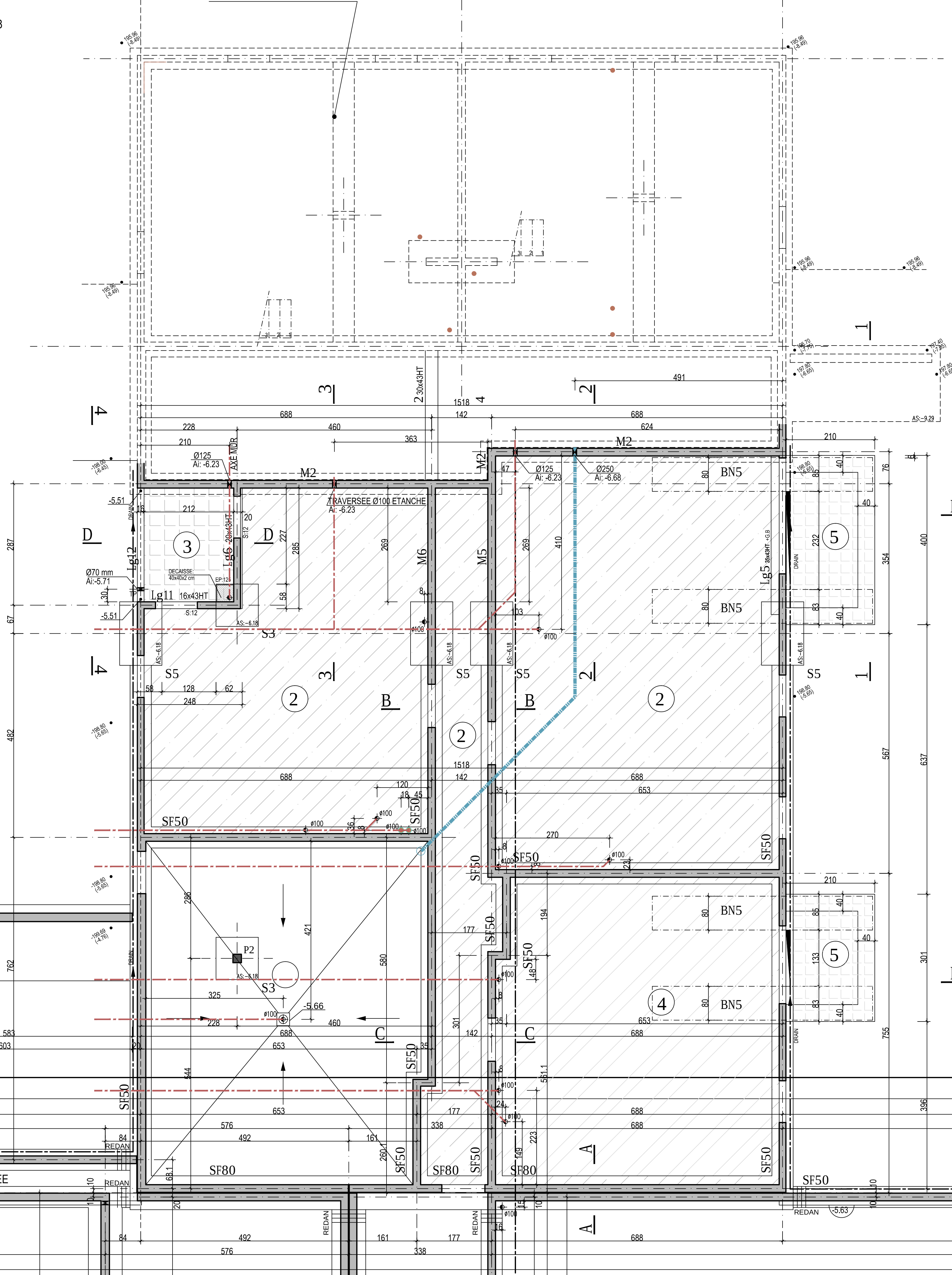
FONDATEURS VOIR PLAN N° C01
