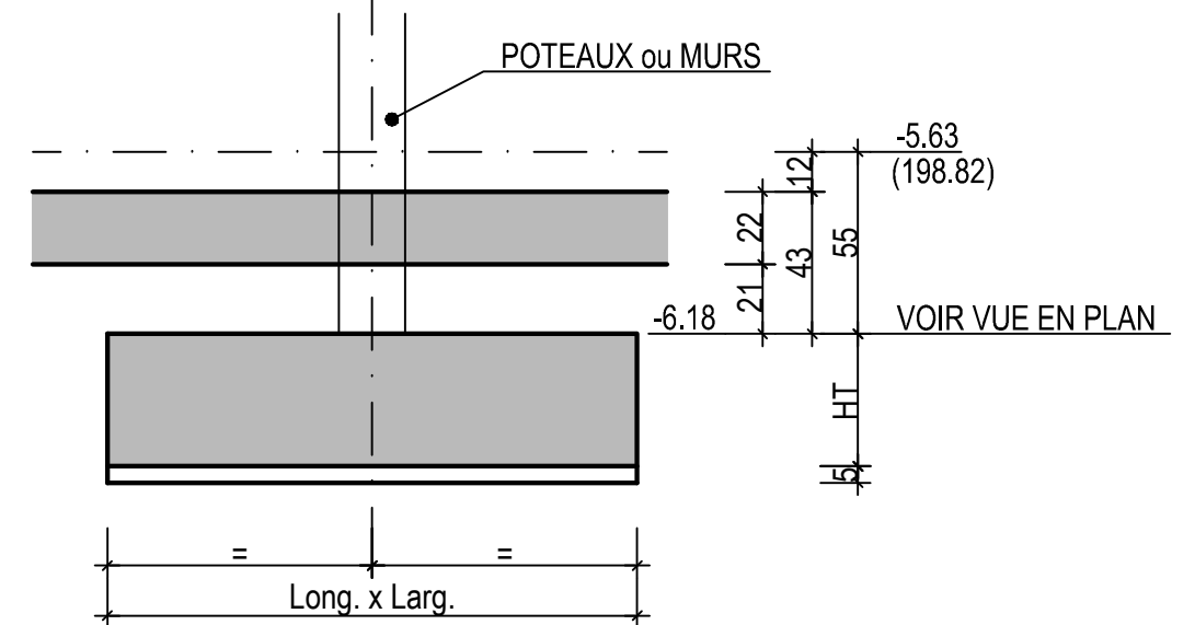
COUPE SUR DALLE
