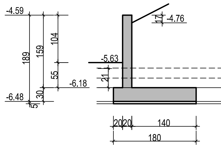
COUPE E Ech: 1/50
