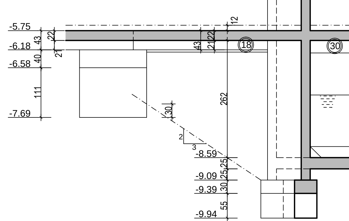
COUPE 1 Ech: 1/50
