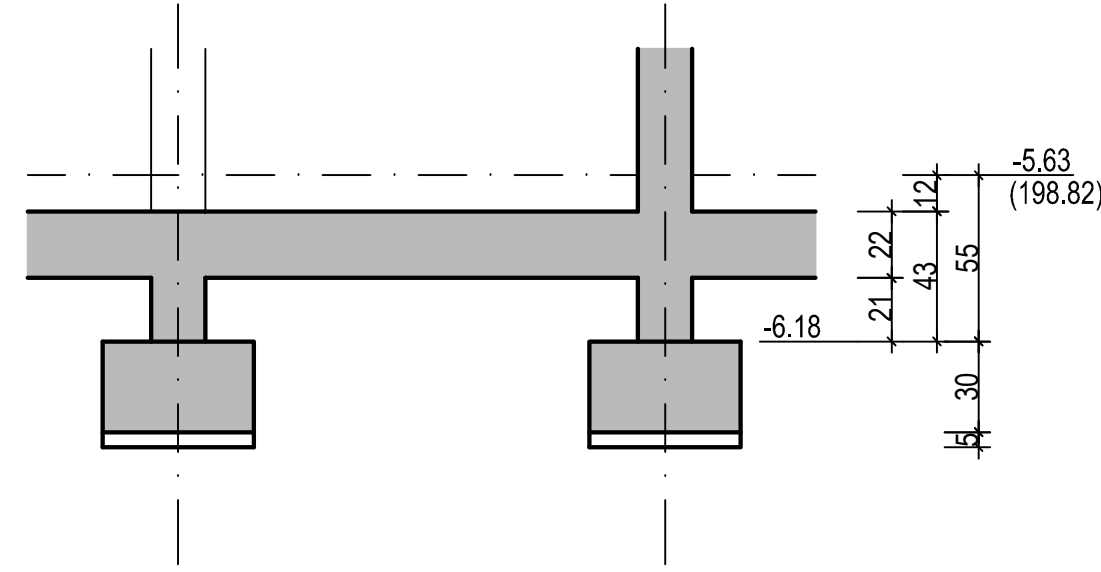
COUPE C Ech: 1/25
