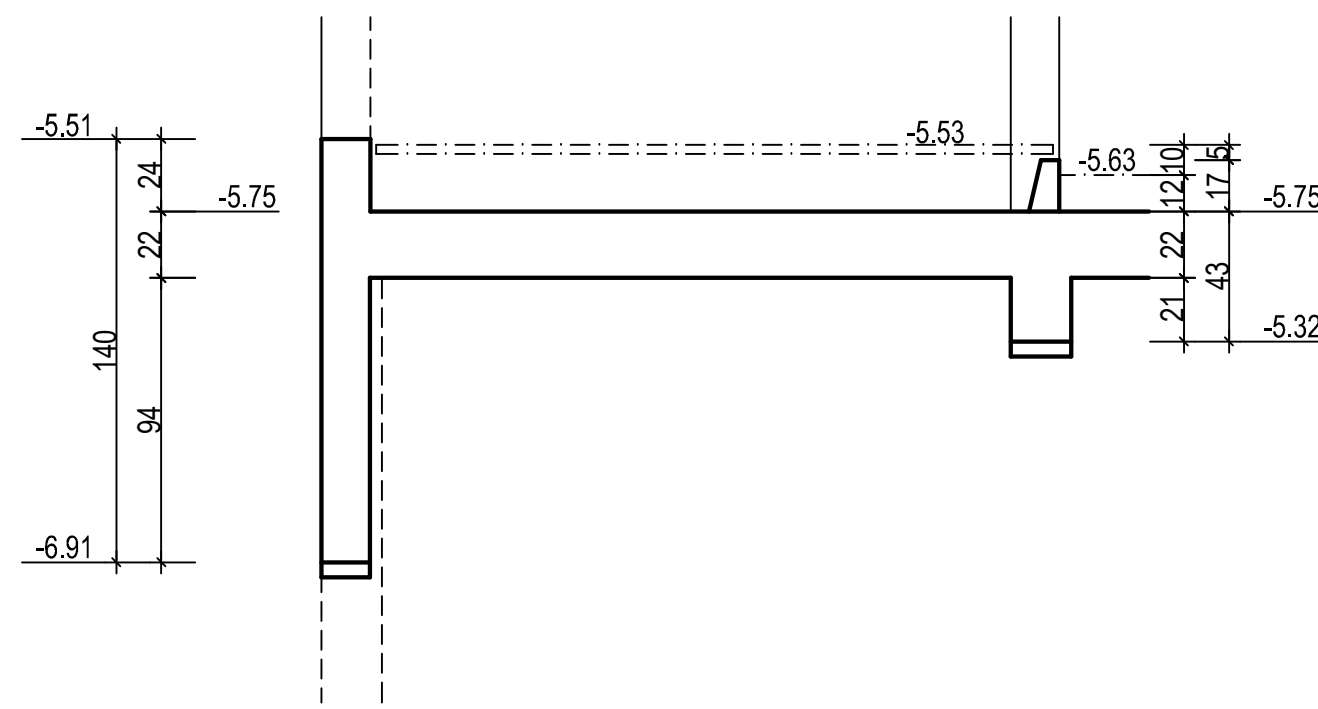
COUPE D Ech: 1/25
