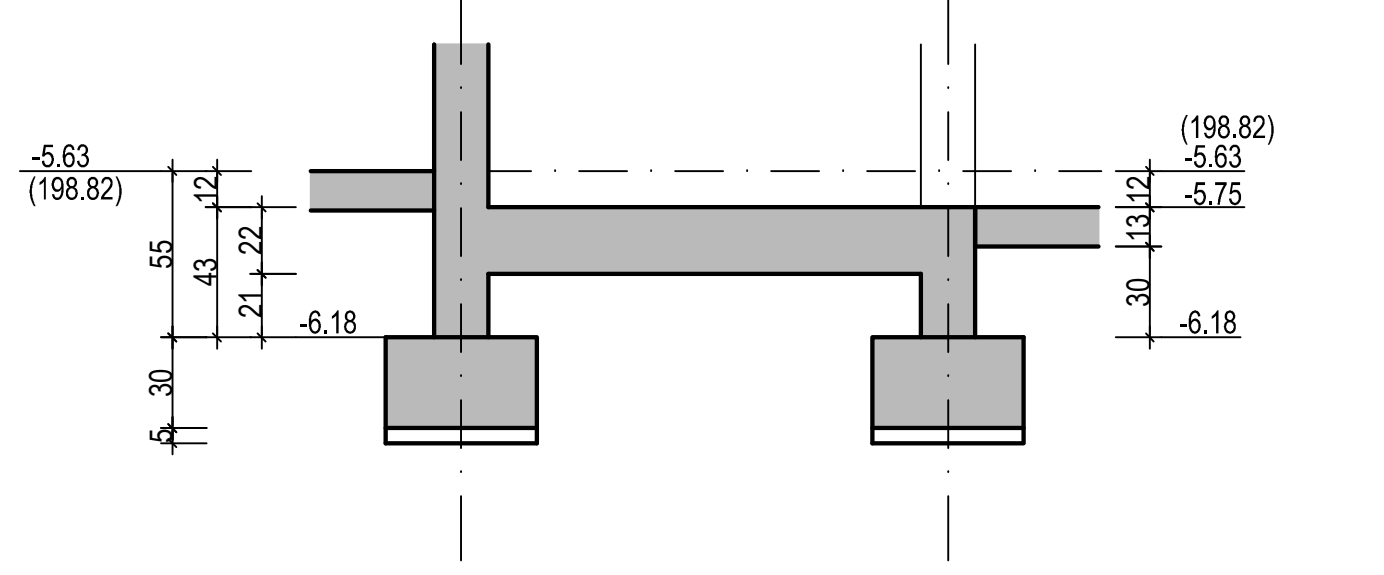
COUPE C Ech: 1/25
